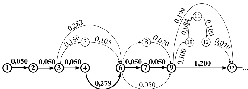
Рис 2. Сетевая модель с выделенным критическим путем
