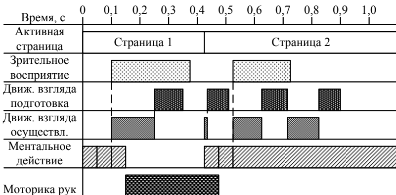
Рис 1. Пример исходных данных – визуализации модели АСТ-R
