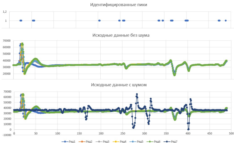
Рис. 1. Идентифицированные пики.
