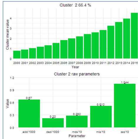
Рис. 6. «Математики»: три кластера без к.п.
