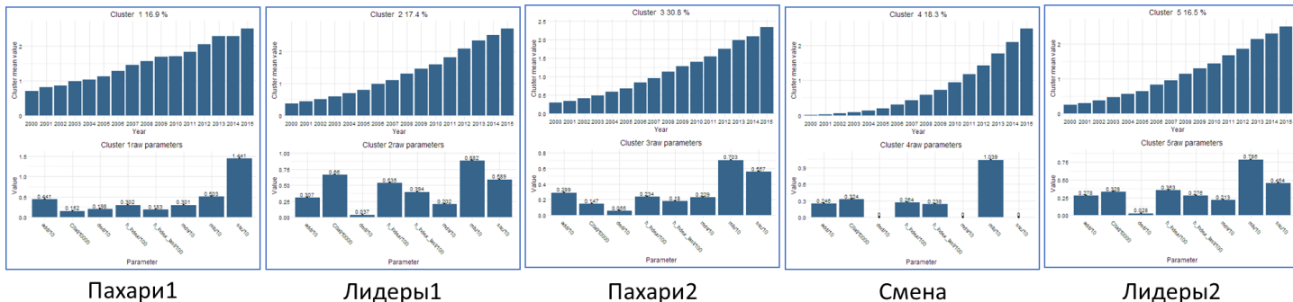
Рис. 29. «Психологи»: пять кластеров
