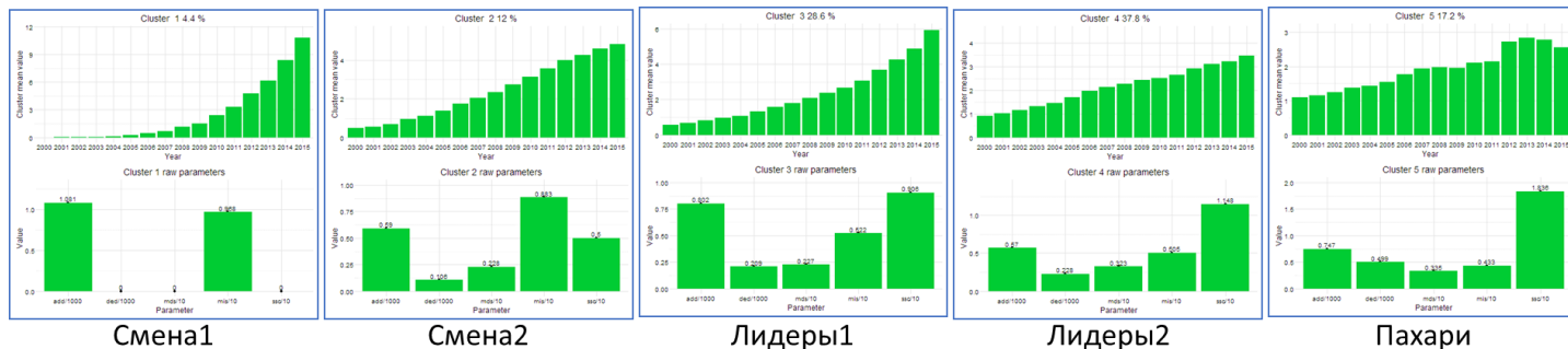
Рис. 8. «Математики»: пять кластеров без к.п.
