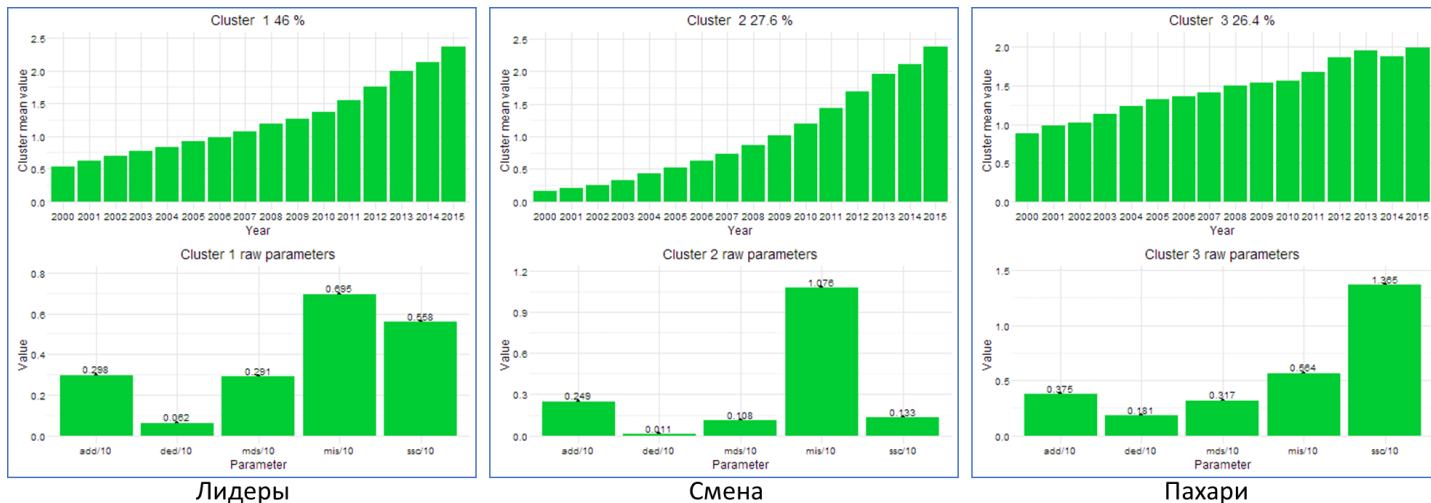
Рис. 19. «Физики»: три кластера без к.п.
