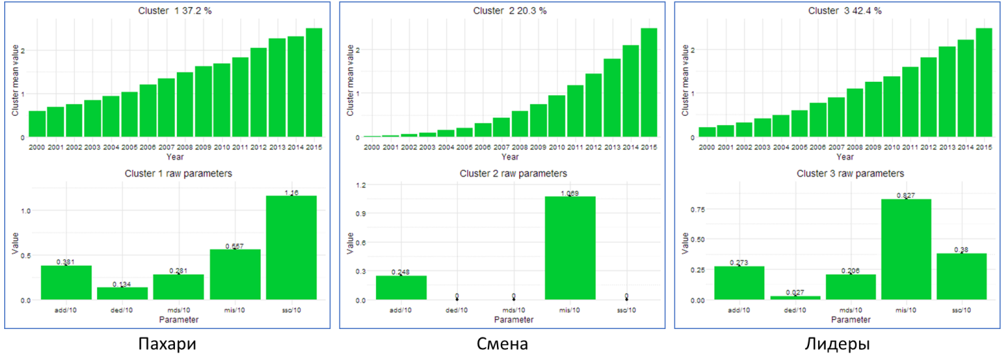
Рис. 27. «Психологи»: три кластера без к.п.
