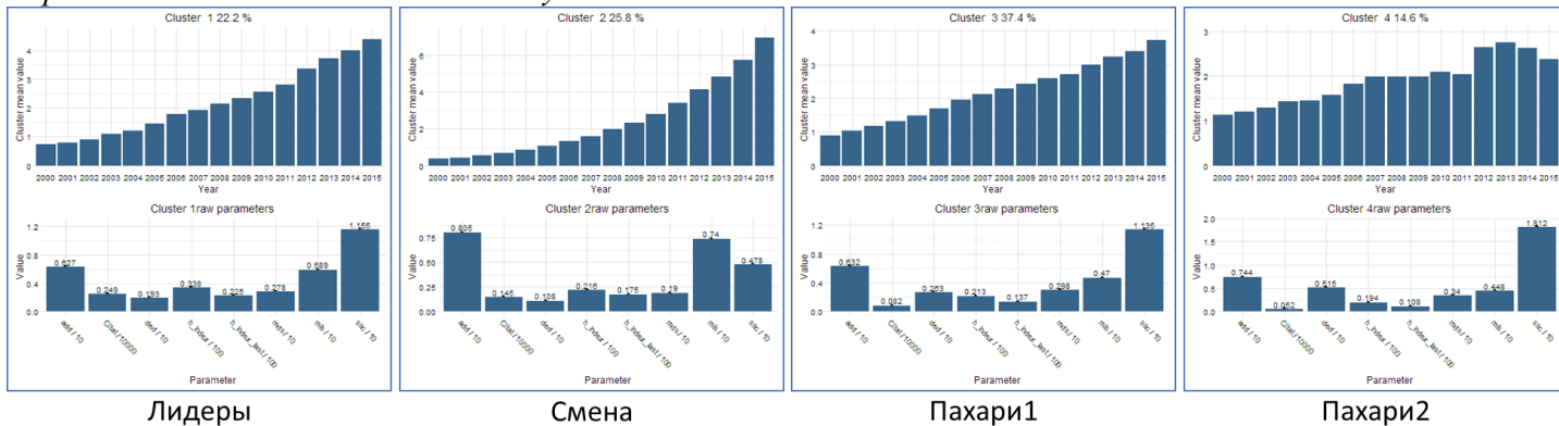
Рис. 3. «Математики»: четыре кластера
