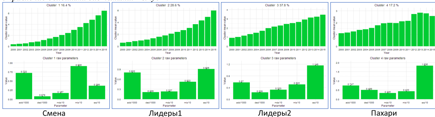
Рис. 7. «Математики»: четыре кластера без к.п.
