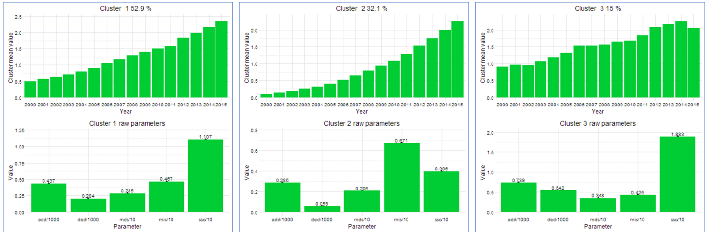
Рис. 11. «Математики+»: три кластера без к.п.
