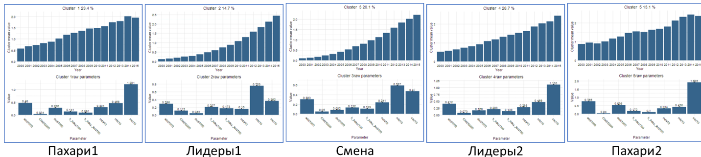
Рис. 13. «Математики+»: пять кластеров
