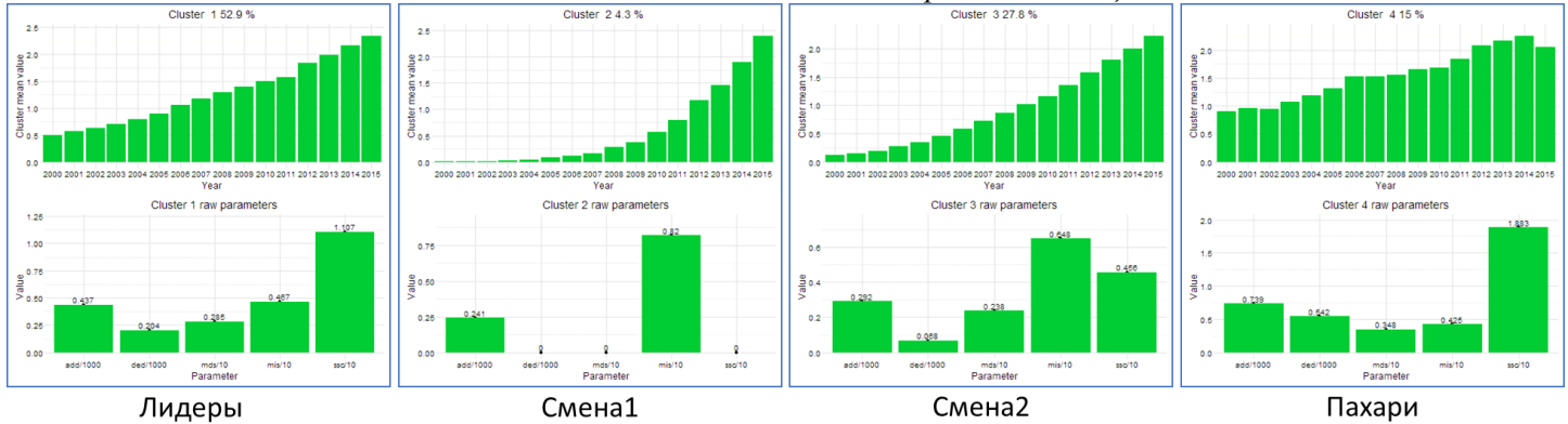
Рис. 15. «Математики+»: четыре кластера без к.п.
