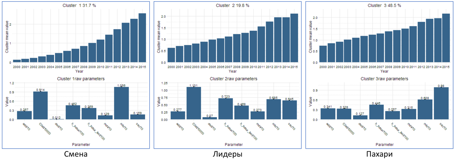
Рис. 18. «Физики»: три кластера
