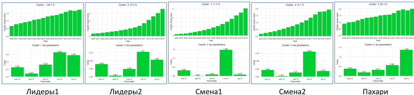
Рис. 24. «Физики»: пять кластеров без к.п.
