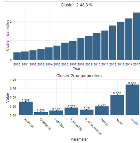
Рис. 10. «Математики+»: три кластера
