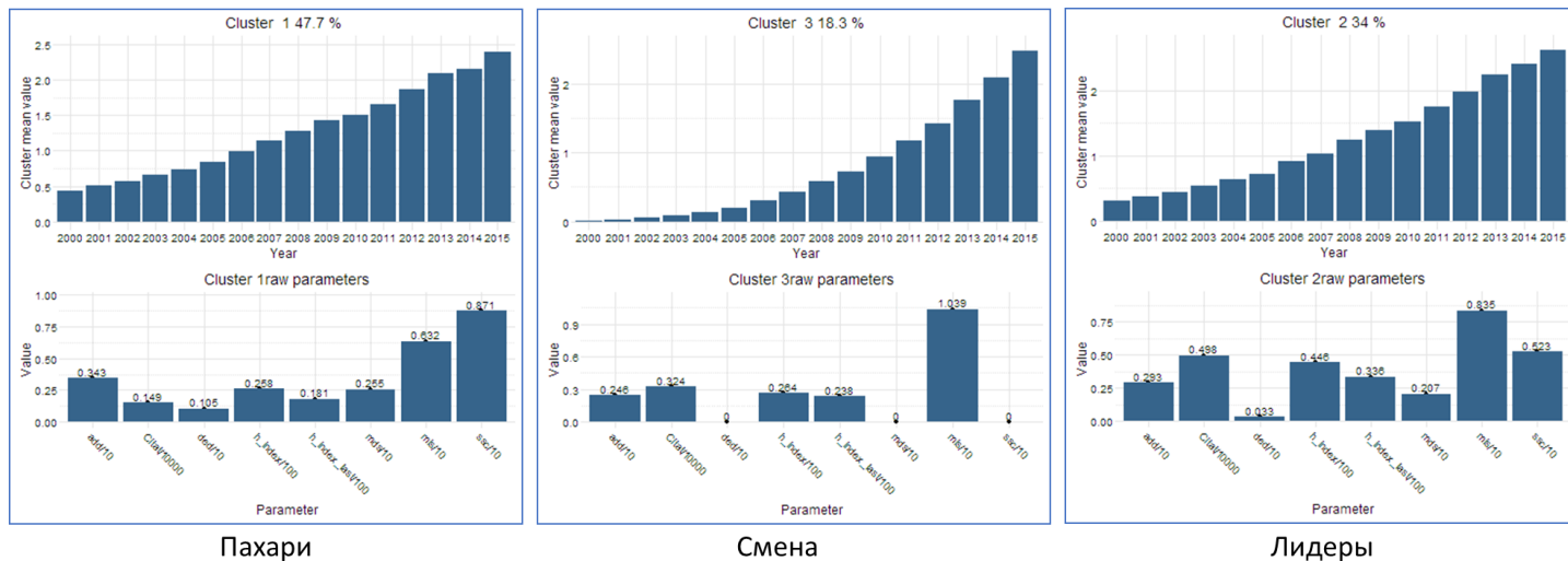
Рис. 26. «Психологи»: три кластера
