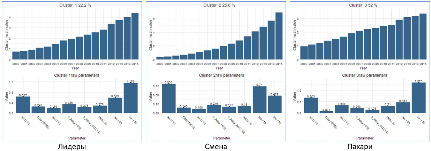
Рис. 2. «Математики»: три кластера
