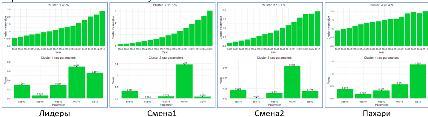
Рис. 23. «Физики»: четыре кластера без к.п.
