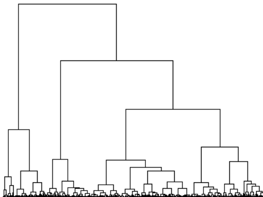
Рис. 1. Пример дендрограммы иерархической кластеризации. Вертикальные линии соответствуют выделенным кластерам
