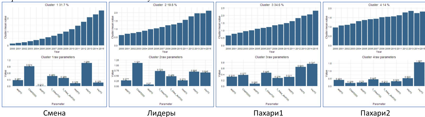
Рис. 20. «Физики»: четыре кластера
