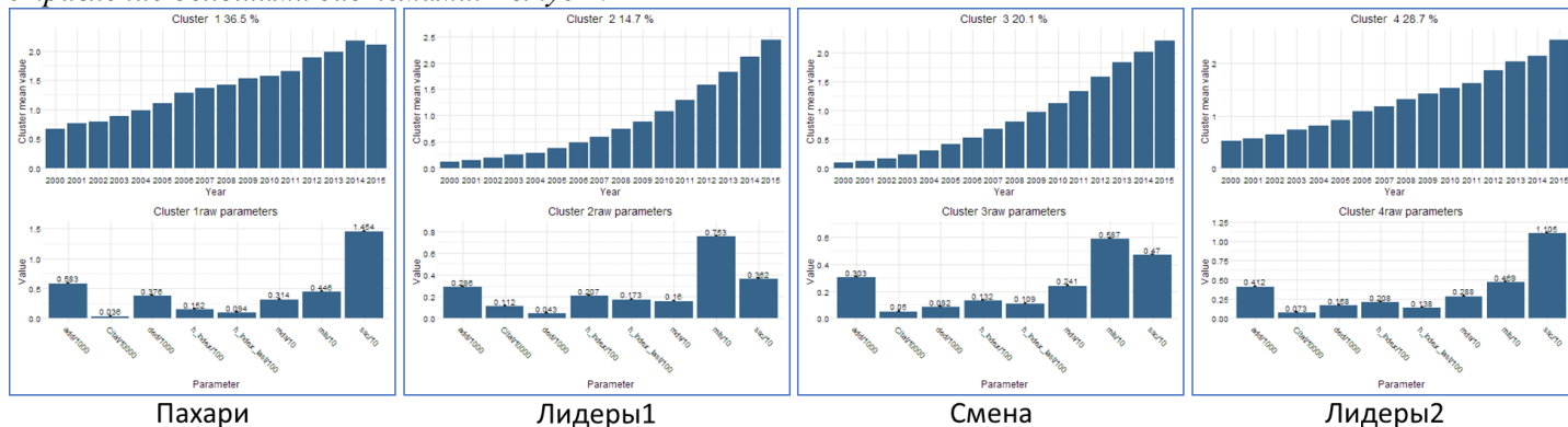
Рис. 12. «Математики+»: четыре кластера
