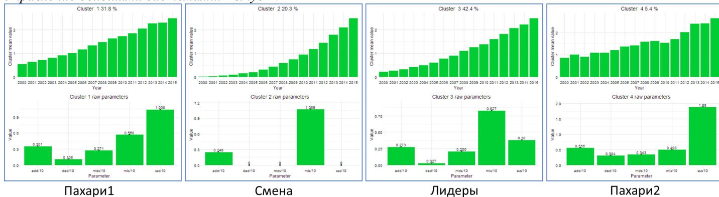
Рис. 31. «Психологи»: четыре кластера без к.п.
